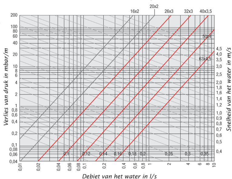
Drukverlies bij 80 °C
